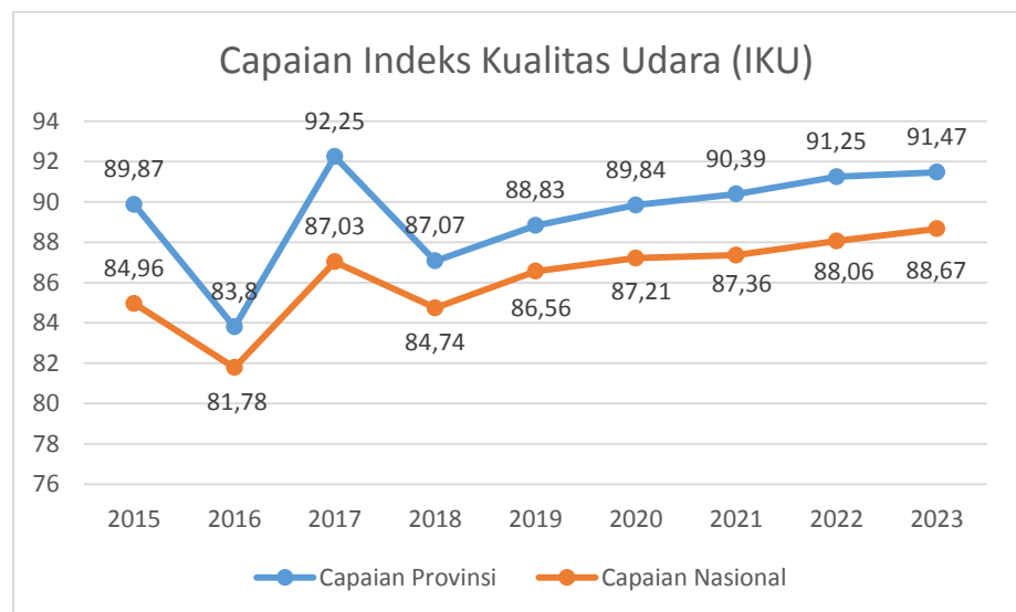
Gambar 2.5 Capaian Indeks Kualitas Udara Tahun 2023
