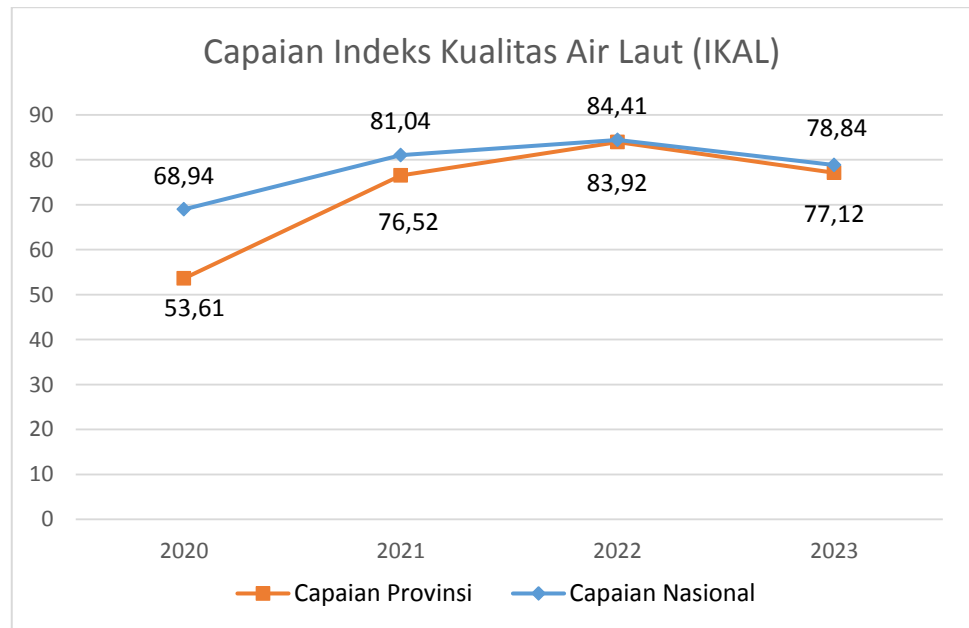
Gambar 2.7 Capaian Indeks Kualitas Air Laut Tahun 2023
