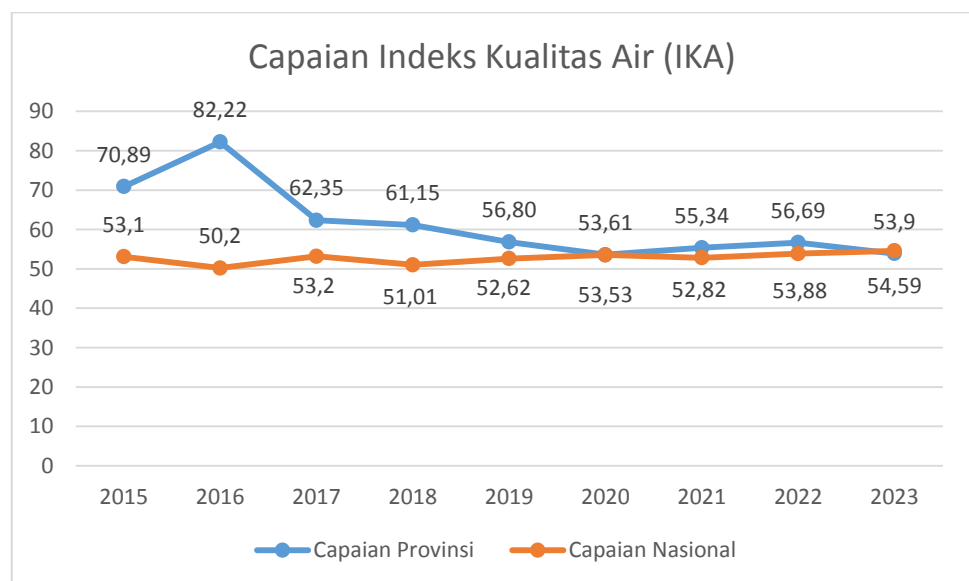
Gambar 2.4 Capaian Indeks Kualitas Air Tahun 2023
