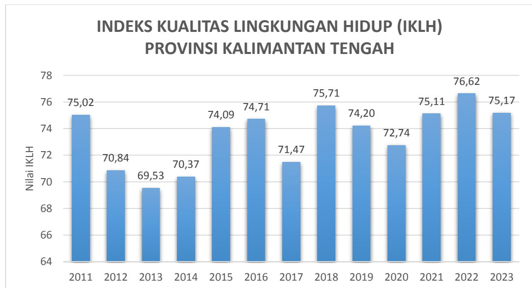
Gambar 2.2 Capaian IKLH Provinsi Kalimantan Tengah
