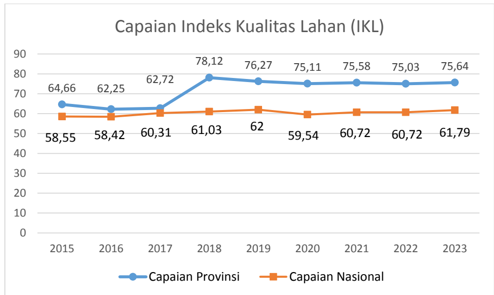
Gambar 2.6 Capaian Indeks Kualitas Lahan Tahun 2023
